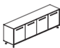
EA96 Ш2400xГ520xВ800 мм Ш1800xГ520xВ800 мм
