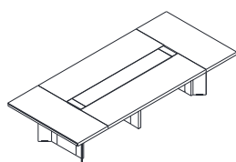
EY78.3400 Ш3400xГ1500xВ750 мм
